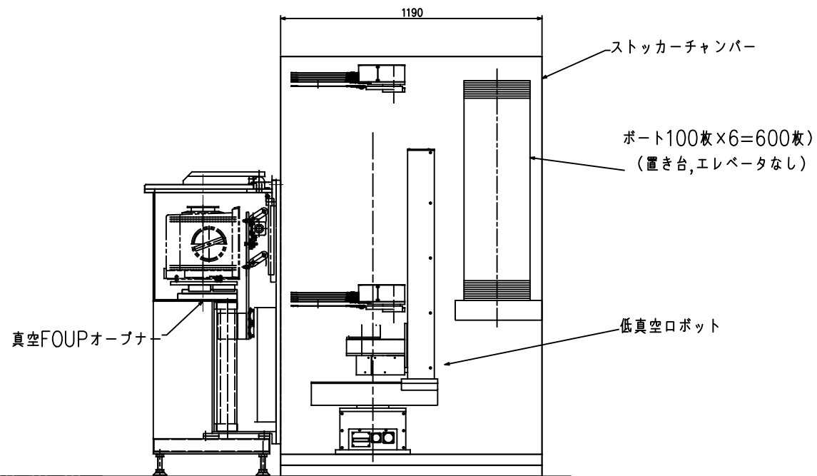
1ポート6ポート 真空ベアウェーハストッカー構想図
