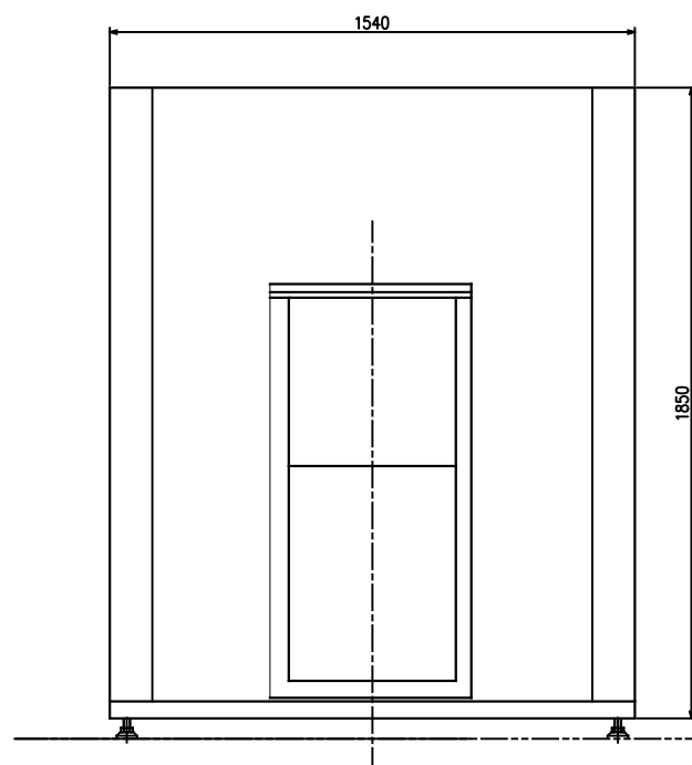
1ポート6ポート 真空ベアウェーハストッカー構想図
