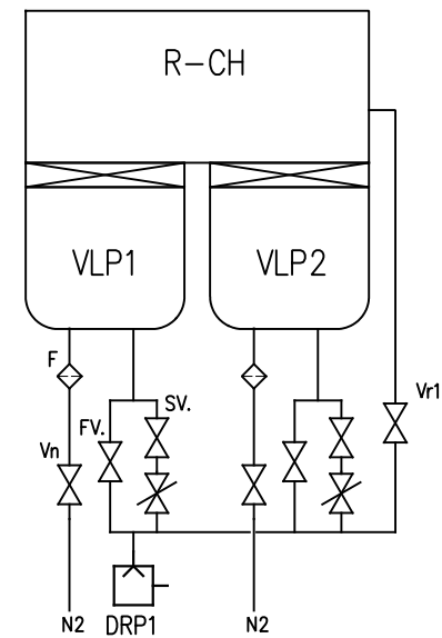
真空およびガス系統図
